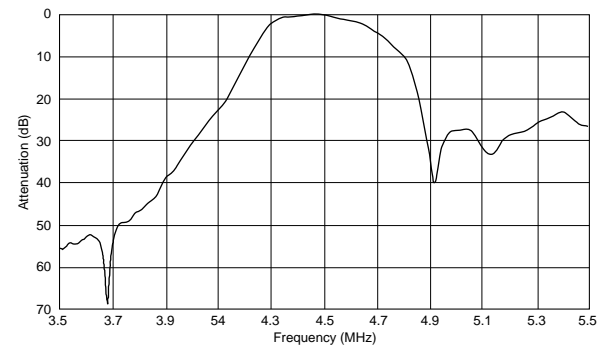
SFSRA4M50EF00-B0
