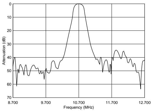
SFECF10M7FA00-R0/SFECF10M7FF00-R0
