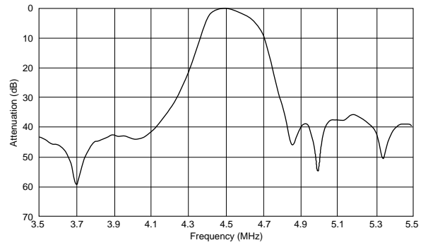
SFSRA4M50CF00-B0
