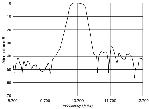
SFECF10M7DA0001-R0/SFECF10M7DF00-R0
