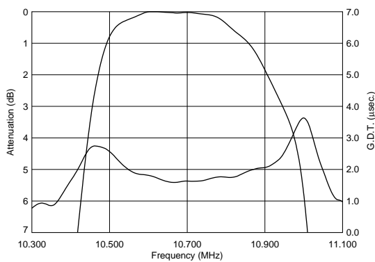
SFECF10M7CQ00-R0
