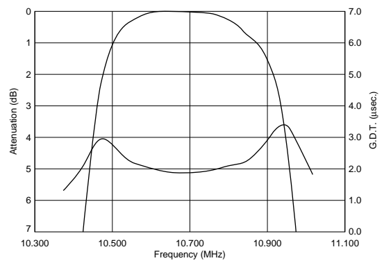
SFECF10M7DF00-R0
