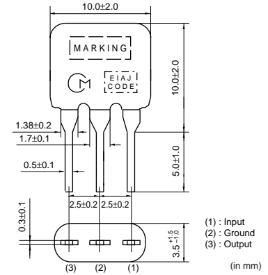
SFKLF10M7NL00-B0
