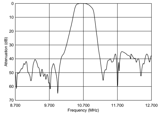
SFECF10M7CQ00-R0
