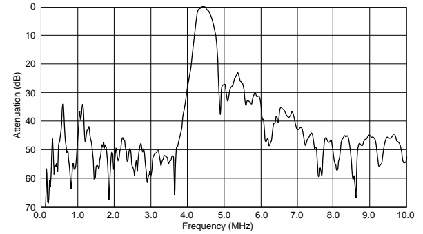
SFSRA4M50EF00-B0
