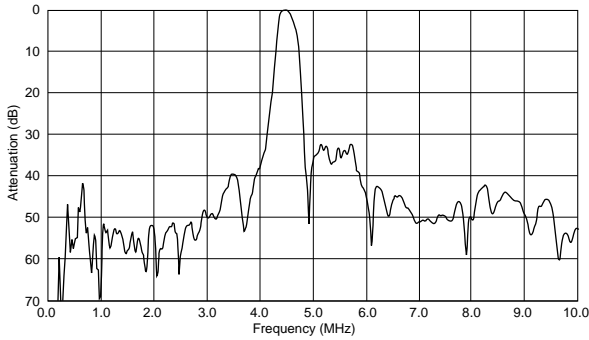
SFSRA4M50DF00-B0
