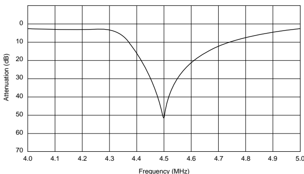
TPSKA4M50B00-R1
